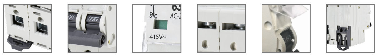
pojemność zacisków: max. 25mm 2 możliwość plombowania kontrolka sygnalizująca zadziałanie możliwość połączenia za pomocą szyn grzebieniowych pole opisowe montaż na szynie DIN35
